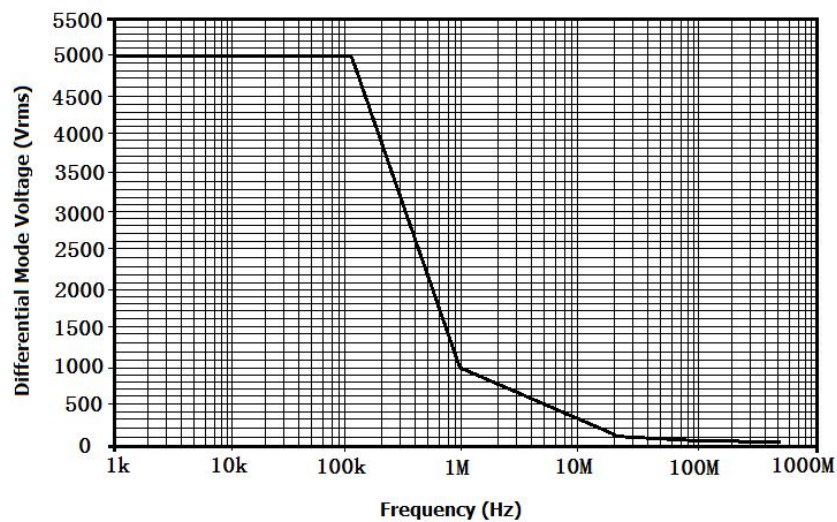
图 3 HVP6700G 最大差模电压 VS 频率
