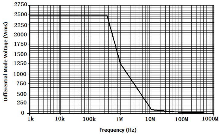
图 2 HVP6350G 最大差模电压 VS 频率
