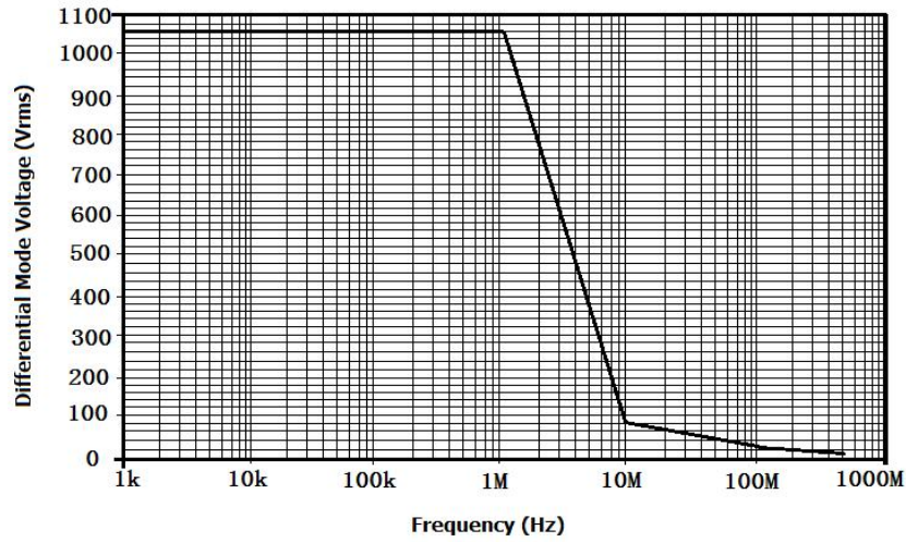
图 1 HVP6150G 最大差模电压 VS 频率
