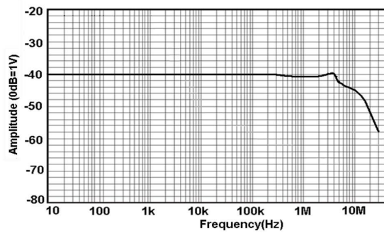
Fig 16 HCPX8500
