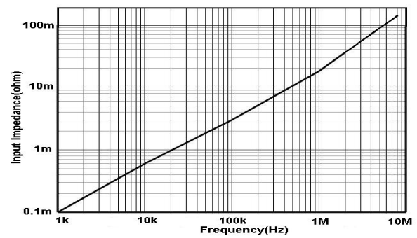
Fig 15.b HCPX8300A
