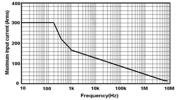
Fig 14.b HCPX8300A
