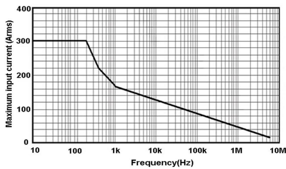
Fig 14.a HCPX8300
