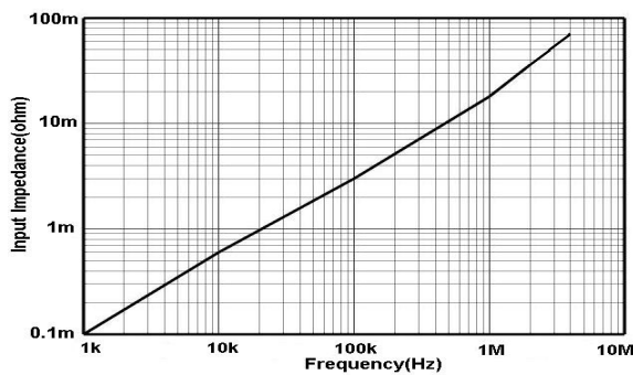
Fig 15 .a HCPX8300
