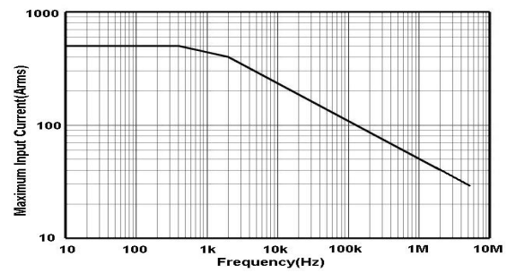
Fig 17 HCPX8500
