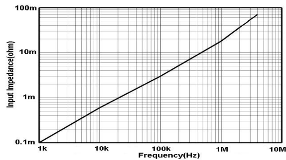
Fig 18 HCPX8500
